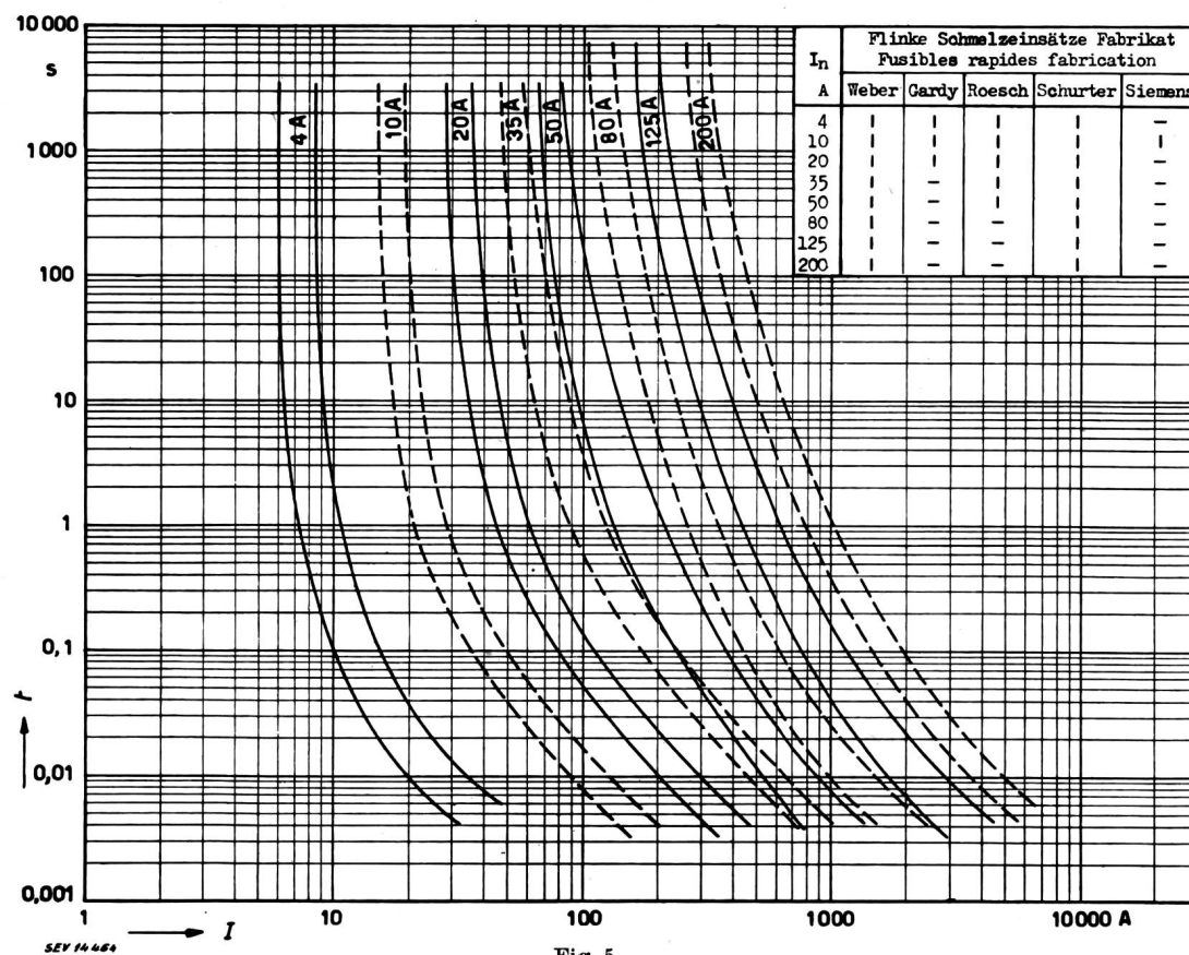
Abschmelzcharakteristik von flinken Schmelzeinsätzen
