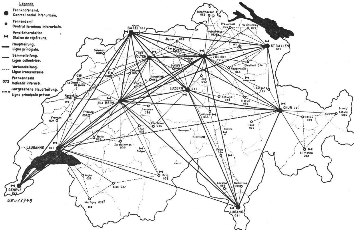
Fig. 8. Automatisches Fernnetz, projektierte Endausbau
