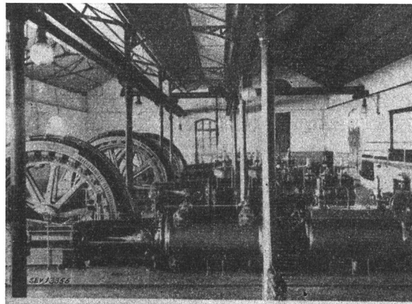
Fig. 5. Zurich-Letten, usine thermique (1896)
