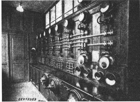
Fig. 3. Usine de Taulan sur Montreux. Le tableau (1887)
