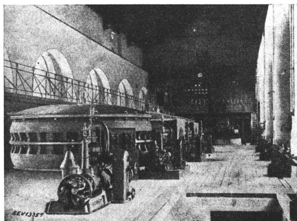
Fig. 7. Genève, usine de Chèvres. Salle des machines (1896)
