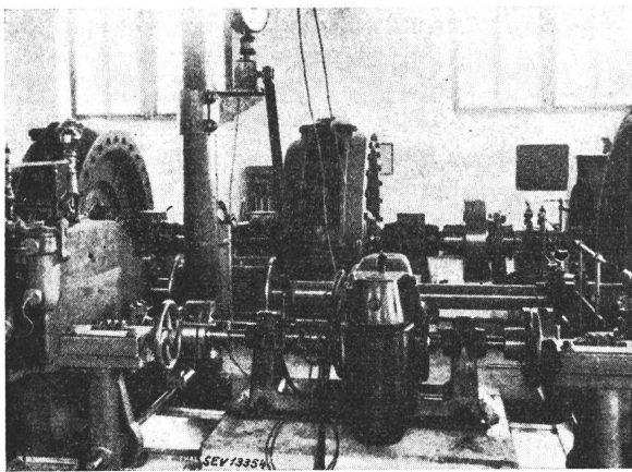
Fig. 4. Zurich-Letten, usine hydraulique (1892)
