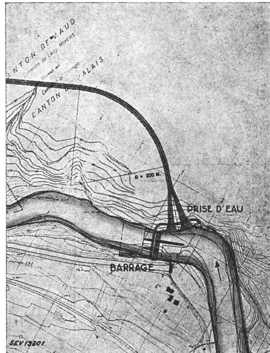
Fig. 2. Barrage et prise d'eau
