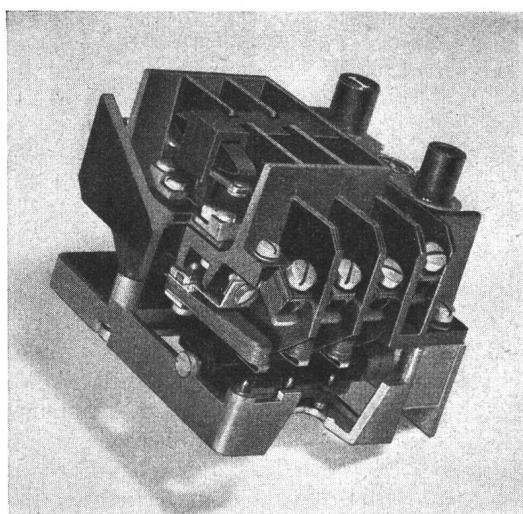
Fig. 3. Kleinmotorschalter Typ KT (ohne Gehäuse)
