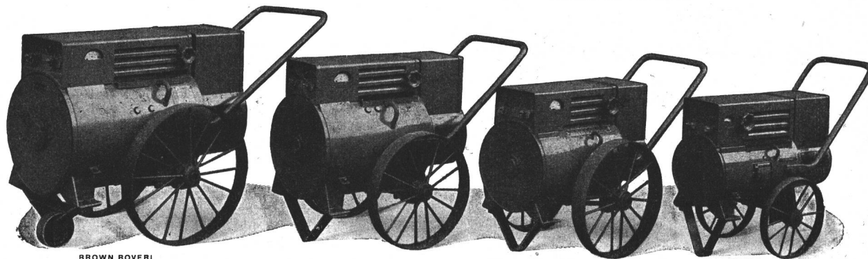
Fig. 2. Brown-Boveri-Gleichstrom-Schweissumformer
