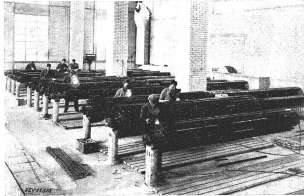
Fig. 7. Schweissen von Betonarmierungsseisen
