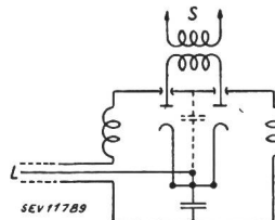
Fig. 8. Ersatzschaltung der Topf- kreisdiode S zum Steuersender. L konzent. Leitung.
