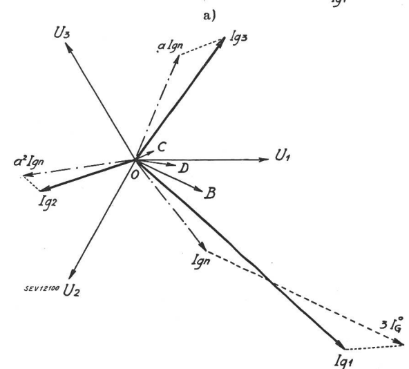
Fig. 3a Diagrammes des courant dans la ligne g a) pour réseau à neutre isolé. b) pour réseau avec bobine d'extinction.
