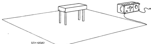
Fig. 3. Störspannungsprüfer, betriebsbereit
