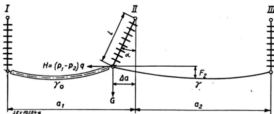
Fig. 1. Freileitung mit ungleich belasteten Feldern a 1 Spannweite mit Zusatzlast a 2 Spannweite ohne Zusatzlast
