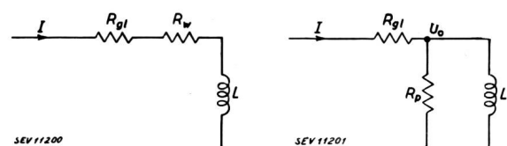
Fig. 1. Fig. 2. Ersatzschema der Massekernspule R_w, R_p Wirbelstromverluste.
