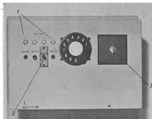
Fig. 4. Piketautomat
