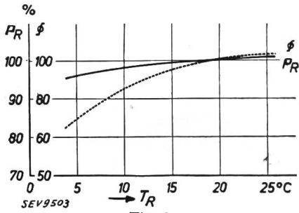
Fig. 9. Abhängigkeit der Leistung (P) und des Lichtstromes (φ) von der Raumtemperatur (T).
