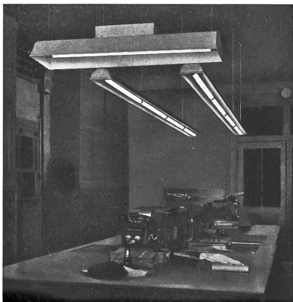
Fig. 15. Schöller & Co., Zürich, Musterraum. In den Reflektoren sind Leuchtstofflampen von 220 V mit tageslichtweisser Farbe eingebaut.
