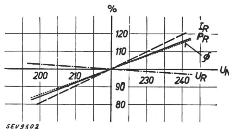
Fig. 8. Abhängigkeit der Leistung (P) und des Lichtstromes ( \Phi ) von der Netzspannung ( U_N ).
