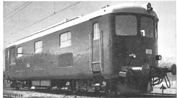
Fig. 3. Dieselelektrische Lokomotive Am 4/4 1001 der SBB. Dauerzugkraft am Radumfang 3090 kg bei 72,5 km/h. Höchstgeschwindigkeit 110 km/h.
