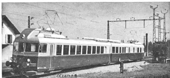
Fig. 1. Leichttriebzug Typ BCFZe 4/6 der BLS. Zugkraft einstündig 3320 kg bei 68,5 km/h. Höchstgeschwindigkeit 110 km/h.
