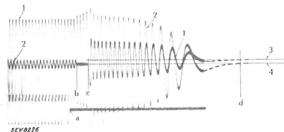
Fig. 9. Oscillogramm der Bremsung eines 440-kW-Synchromotors zum Antrieb einer Gummi-Walzenstrasse. Zeitmaßstab: 50 Hz = 1 Sekunde, 5 Hz = 1 Umdrehung.
