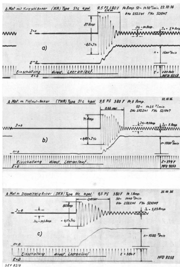
Fig. 3. Leeranlauf.
