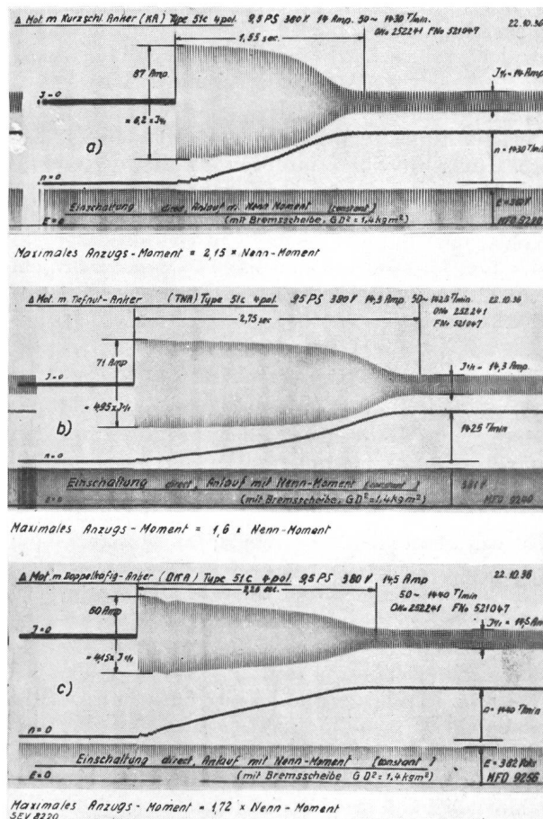
Maximales Anzugs-Moment = 1,72 x Nenn-Moment
