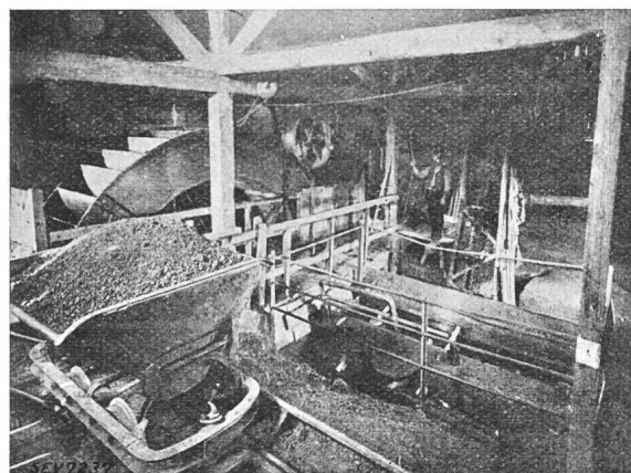
Fig. 12. Bohnerz-Bergbau: Erzwäsche.
