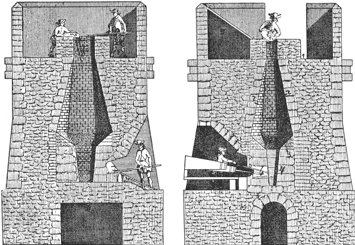
Fig. 20. Holzkohle-Hochofen.
