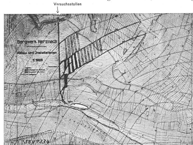
Fig. 17. Bergwerk Herznach: Abbau- und Installations-Plan. ■ Abgebaut bis 1. Februar 1938. ▨ Zum Abbau vorgesehen. / Isohypsen. Aequidistanz 5 m. Der Abbau erfolgt zwischen den Isohypsen 460—465—470 m ü. M.
