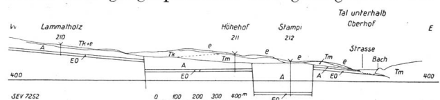
Fig. 10. Querprofil durch das Schollengebiet von Wölflinswil. Y Bohrung. A Argovien. EO Eisenoolith. e (Erraticum-)Grundmoräne. Tm Rote Mergel (mit Juranagelfluh). (Nach Dr. A. Amstler.)
