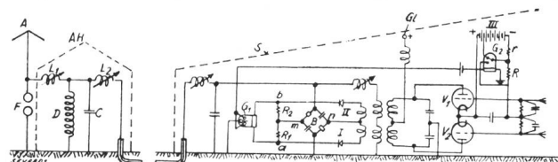
Fig. 1. Anordnung der Schnellabschaltung. A Antenne, AH Abschirmhülle, S Senderhaus, G1 vom Gleichrichter.
