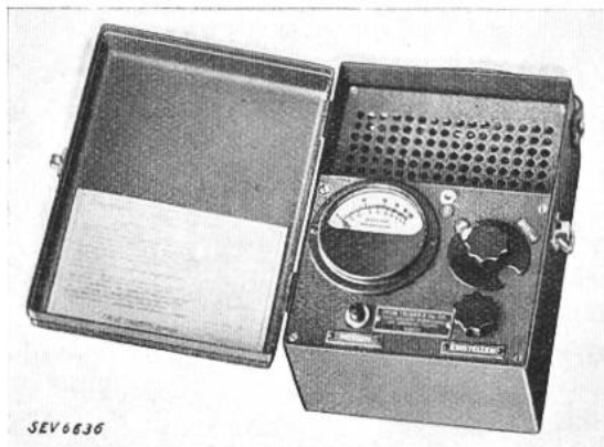
Fig. 5. Erdungsprüfer für 145, 220 und 290 V Netzspannung.
