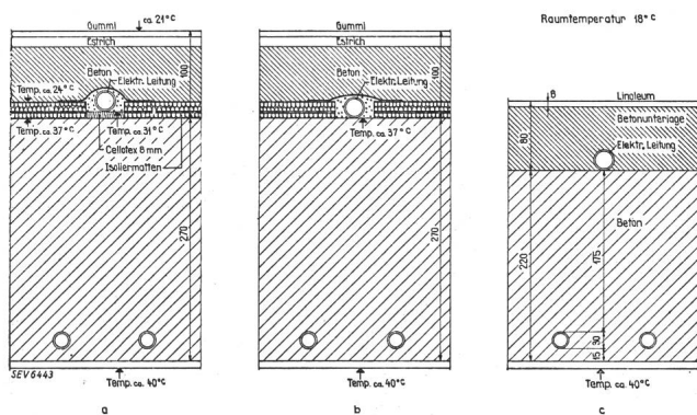
Fig. 1. Verschiedene Bodenbauarten mit Deckenheizung.
