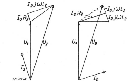
Fig. 2. Spannungs-Diagramme. Einphasen-System (links) und Dreiphasen-System (rechts).
