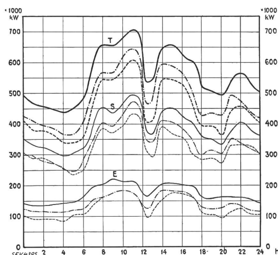
Fig. 9. Belastungsverlauf an je einem Junimittwoch der Jahre 1932, 1933 und 1934.
