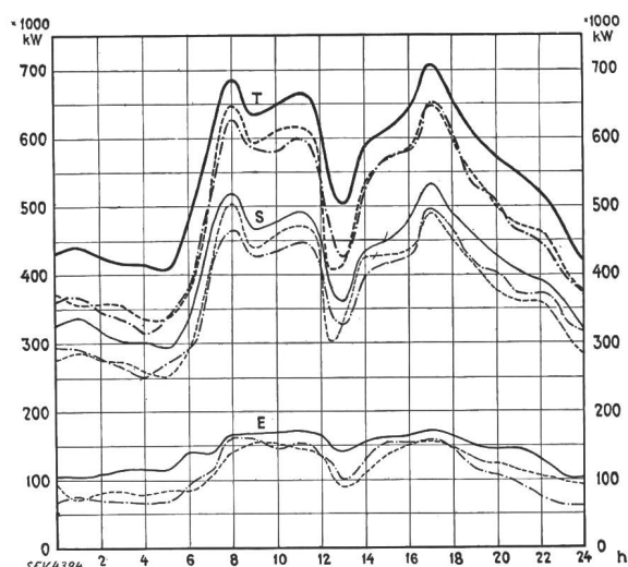
Fig. 8. Belastungsverlauf an je einem Dezembermittwoch der Jahre 1931, 1932 und 1933.
