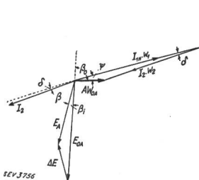
Fig. 2. Stromwandlerdiagramm für Auslösung.
