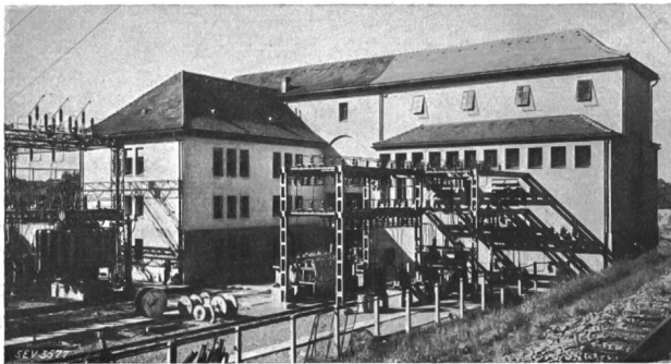
Fig. 18. Ansicht der Gebäulichkeiten des Unterwerkes mit den Drehstromfreiluftanlagen.
