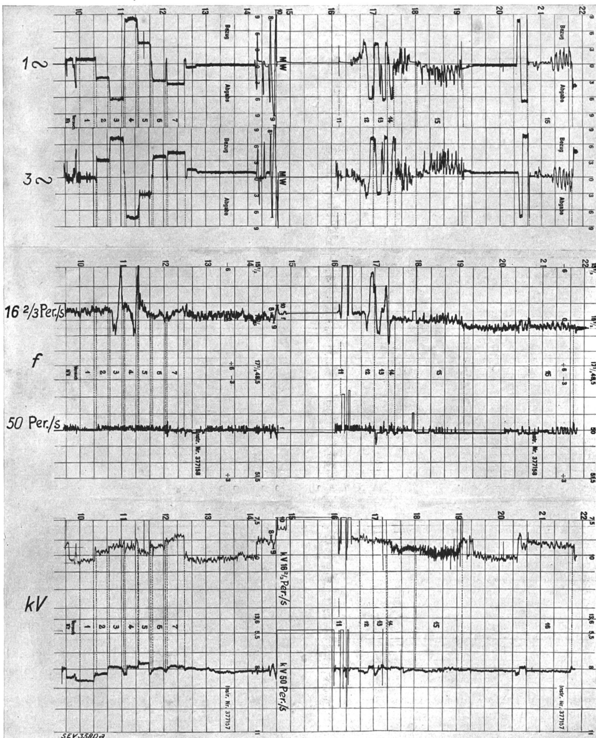
Fig. 21. Betriebsdiagramme.
