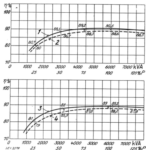
Fig. 19. Wirkungsgradkurven der Frequenzumformergruppe mit Reguliereinrichtung bei Energieübertragung von NOK nach SBB.
