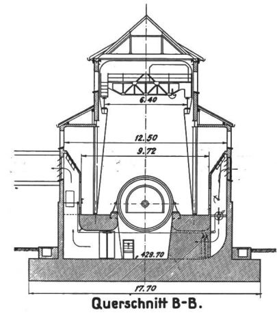
Fig. 17. Grundriss der Anlage. Längs- und Querschnitte durch das Maschinenhaus.
