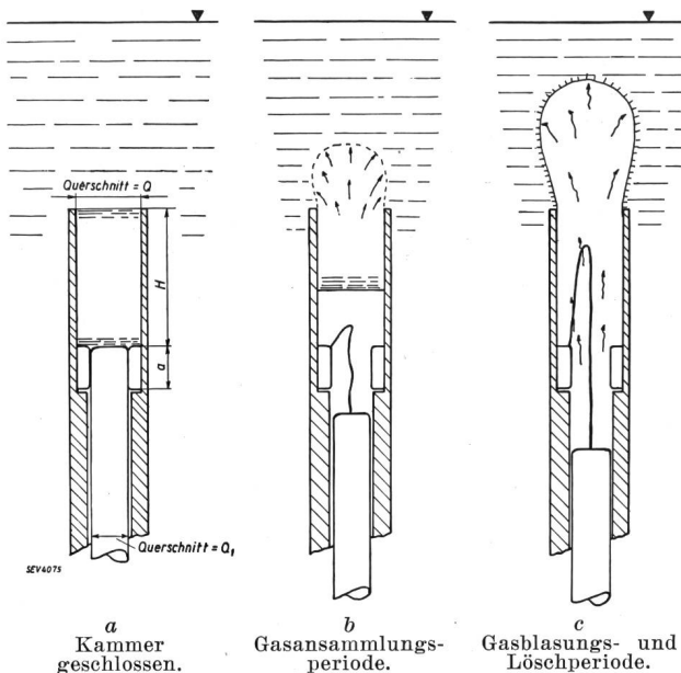
Fig. 4. Arbeitsweise des Schalters.
