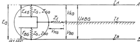
Fig. 9. Unsymmetrisch belasteter Einphasengenerator.
