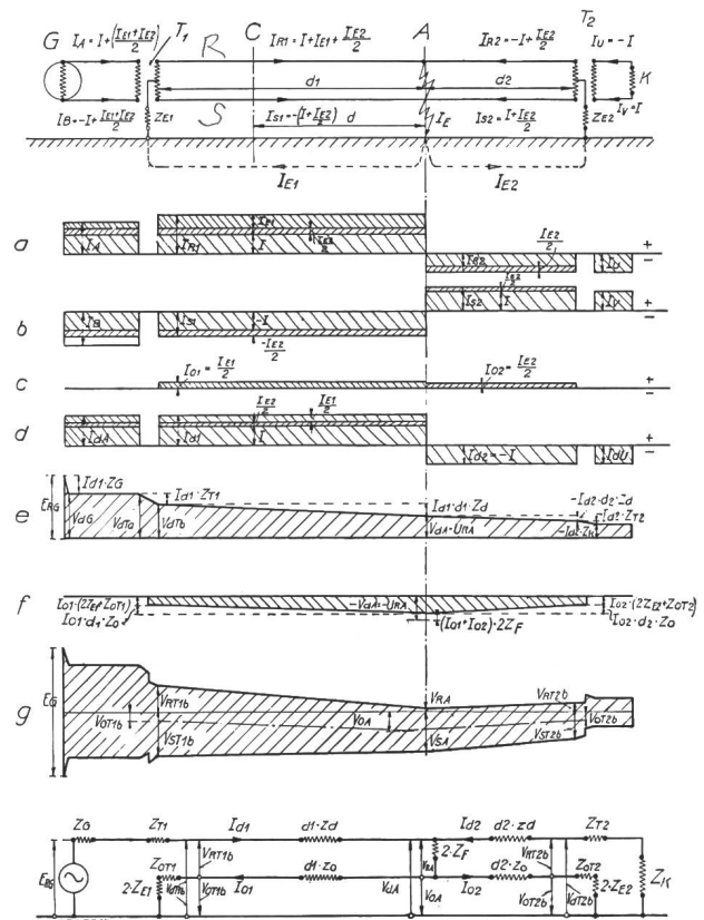
Fig. 2. Der Erdschluss im Einphasennetz mit Nullpunktterdung über Impedanzen. Räumlicher Verlauf a der Ströme in Phase A—R—U b der Ströme in Phase B—S—V c der Nullstromkomponente d der Schleifenstromkomponente e der Phasen-(Schleifen)Spannung f der Nullspannung g der Spannungen gegen Erde Ersatzschaltbild der Bezugsphase.
