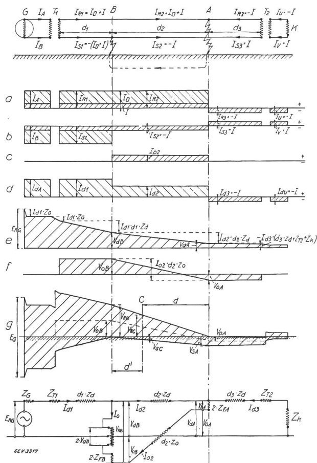
Fig. 5. Der Doppelerdschluss im isolierten Einphasennetz.
