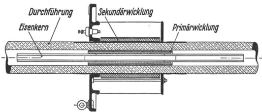
Fig. 1. Eisenstabwandler. Schematischer Aufbau.
