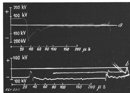
Fig. 4. Oszillogramme der Blitzstörung No. 5 in Tab. II, vom 5. VIII., 15 h 39. Fig. 4a ist gemessen in Phase BV (Fig. 6). Fig. 4b ist gemessen in Phase BU (Fig. 6).
