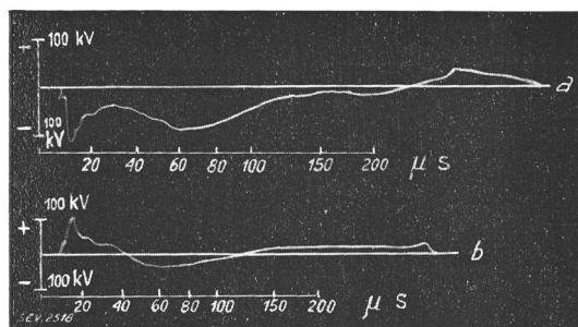
Fig. 8. Oszillogramme der Blitzstörung No. 1 in Tab. II, vom 24. VI., 19 h 38. Fig. 8a ist gemessen in Phase BU (Fig. 3). Fig. 8b ist gemessen in Phase AV (Fig. 3).
