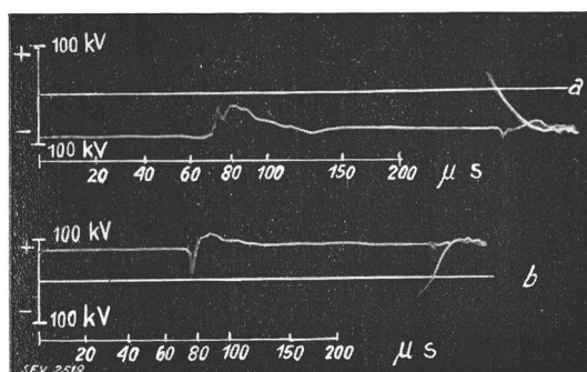
Fig. 9. Oszillogramme einer Ueberspannung infolge eines Blitzes über der Leitung nach Fig. 3, vom 17. VI., 23 h 03. Fig. 9a ist gemessen in Phase BU (Fig. 3). Fig. 9b ist gemessen in Phase AV (Fig. 3).
