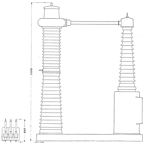
Fig. 7. Grössenverhältnis des kleinsten und grössten Expansionschalters.
