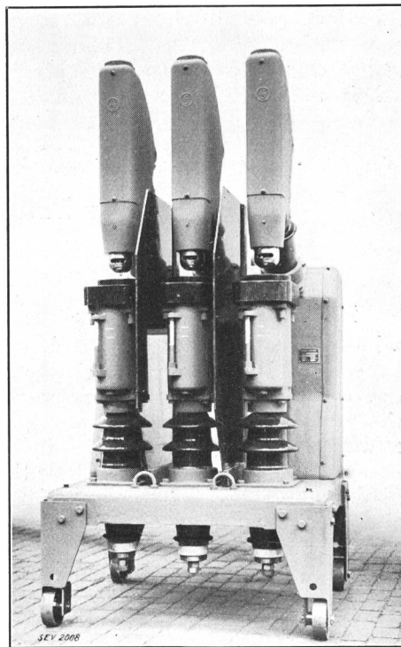
Fig. 9. Expansionschalter 10 kV, 600 A, Abschaltstromstärke 30 kA.
