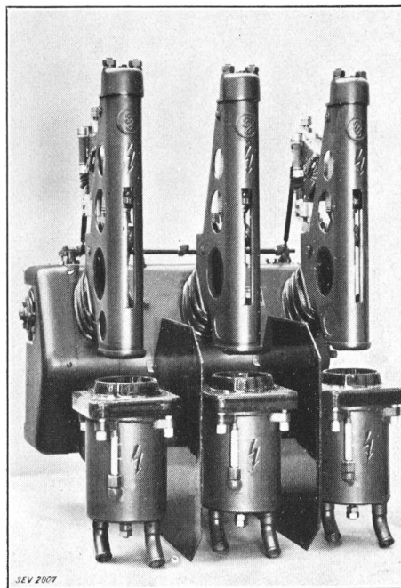
Fig. 8. Expansionschalter 10 kV, 350 A, Abschaltstromstärke 15 kA.
