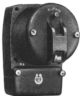
Fig. 4. Automatischer Hausanschlusskasten.
