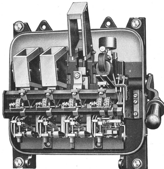
Fig. 5. Stationsschutzschalter.
