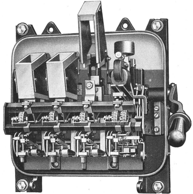
Fig. 5. Stationsschutzschalter.
