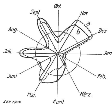
Fig. 24. Anzahl Störungen und betroffene Spannungsklassen pro Monat 1928
