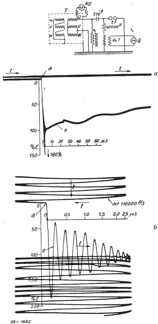
Fig. 13. Kathodenstrahlzillogramm der Spannung zwischen Klemme U und Erde bei Stossprüfung nach Fig. 3. Ueberschwingen der Klemmenspannung bis 180% d.E. C = 7 \cdot 10^{-9} F, R = 100\ 000 Ohm, r = 50\ 000 Ohm. Pr.T = Prüftransformator. Hochfrequenzschwingung mit f = 4,2 \cdot 10^6 Per/s.
