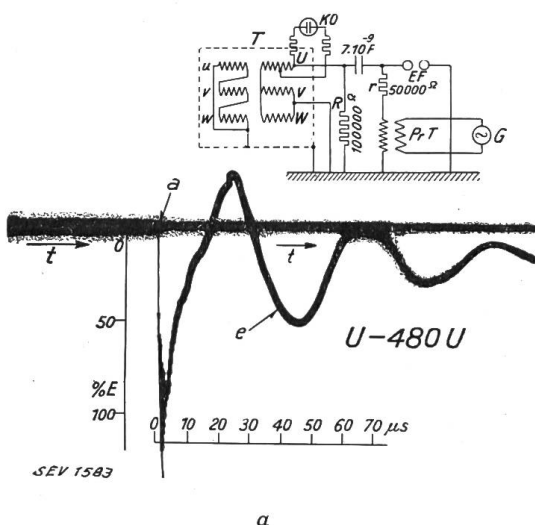
Fig. 14. Kathodenstrahlzillogramm der Spannung über die 1. Doppelspule ( U-480 U ) bei Prüfung nach Schaltung Fig. 3 R = 100\ 000 Ohm, r = 50\ 000 Ohm, C = 7 \cdot 10^{-9} F.
