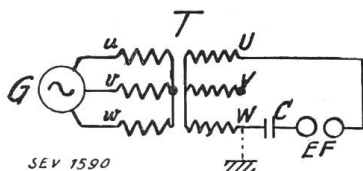
Fig. 21. Anordnung zur Sprungwellenprobe nach VDE-Methöde.
