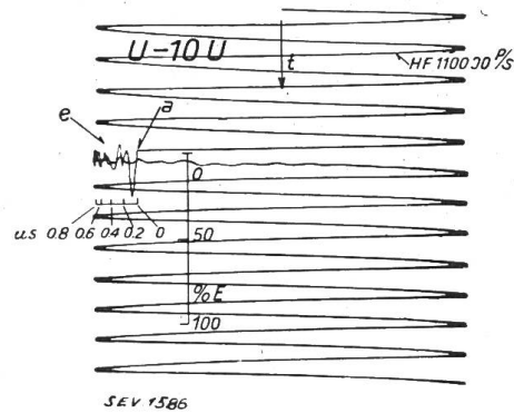
Fig. 17. Wie Fig. 14. Spannung über die ersten 10 Windungen U-10 U.
