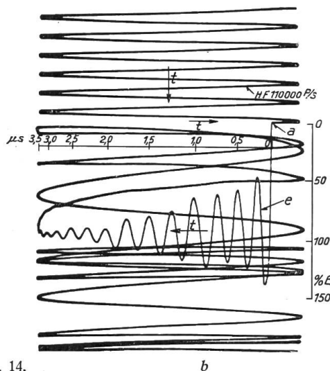
Fig. 14. Kathodenstrahlzillogramm der Spannung über die 1. Doppelspule ( U-480 U ) bei Prüfung nach Schaltung Fig. 3 R = 100\ 000 Ohm, r = 50\ 000 Ohm, C = 7 \cdot 10^{-9} F.
