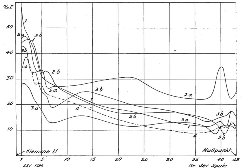
Fig. 20. 3 Phasen-Transformator, 6000 kVA, 45 kV. Spulenbeanspruchung bei verschiedenen Prüfmethöden.
