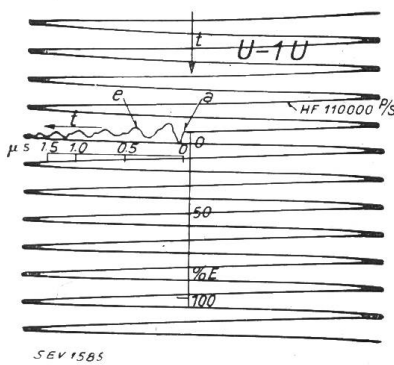
Fig. 16. Wie Fig. 14. Spannung über die 1. Windung U-1 U.
