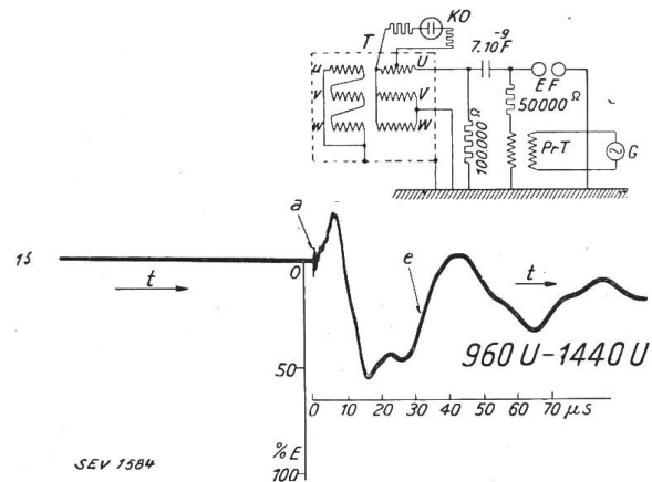
Fig. 15. Wie Fig. 14. Spannung über die letzte Doppelspule (960 U - 1440 U).
