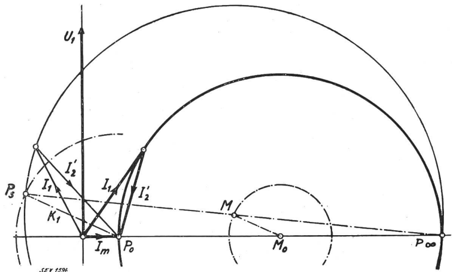
Fig. 4. Drehstrommotor mit fremderregtem Kompensator.
