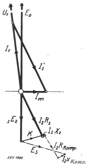
Fig. 3. Drehstrommotor mit fremderregtem Kompensator.
