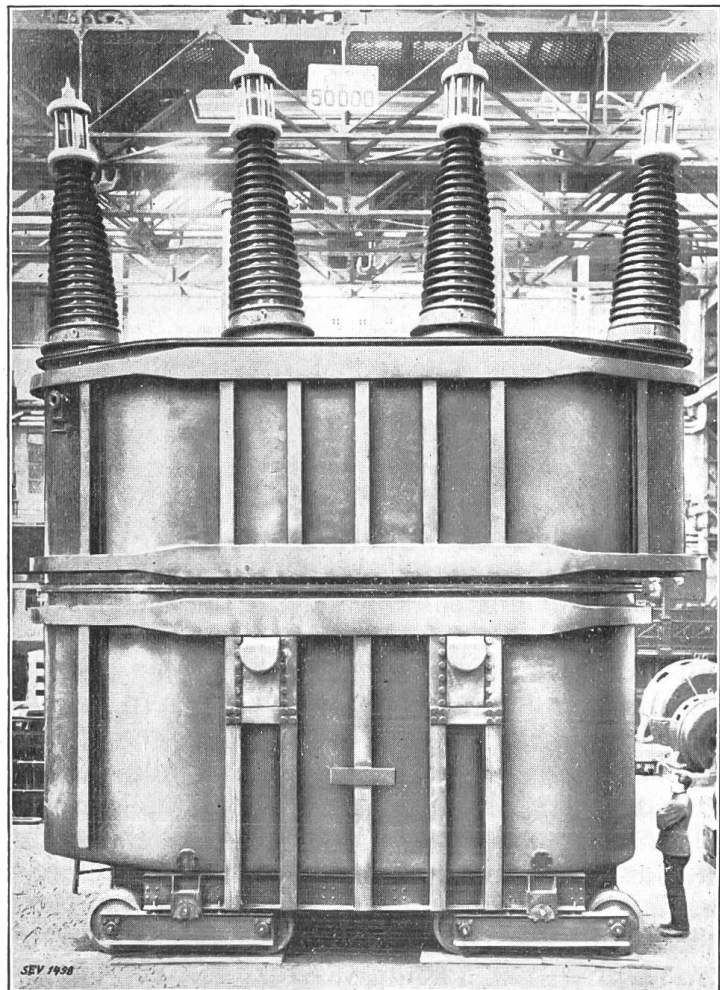
Fig. 3. Drehstromtransformator für Freiluftaufstellung mit Oelumlaufl und Wasserkühlung, 36 000 kVA, 42 und 50 Per s, 11/252 kV. Geteilter Oelkasten. Oelkonservator abmontiert.
