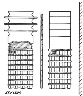
Fig. 2. Schutzring, der Oberspannungswicklung vorgeschaltet.
