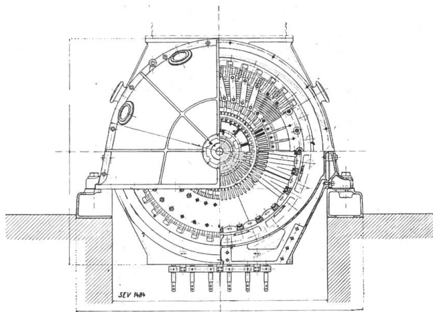
Fig. 2. Dreiphasen-Generator 45000 kVA, 3000 U/m für das Kraftwerk Laziska, Gorne (Polen).
