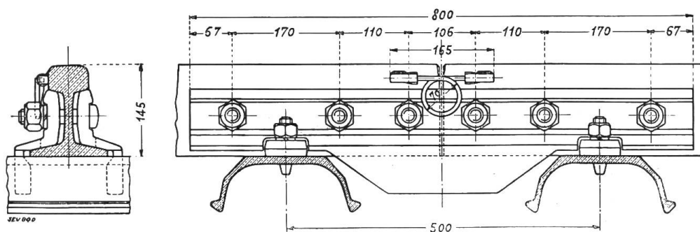
Fig. 4. Éclisse électrique.
