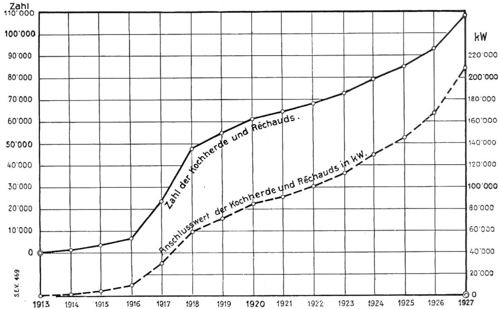
Fig. 3. Stand der Anschlüsse von Kochherden und Réchauds in der Schweiz nach Zahl und Anschlusswert je auf Ende der Jahre 1913 bis 1927. (Ende 1913: Zahl: 600, Anschlusswert: 910 kW.)
