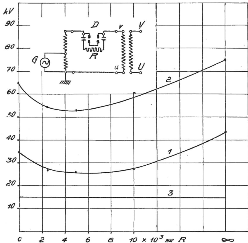
Fig. 25. Surtensions de déclenchement d'un transformateur de 3000 kVA, 15/60 kV, 16,66 p:s, en fonction de la résistance de choc.
