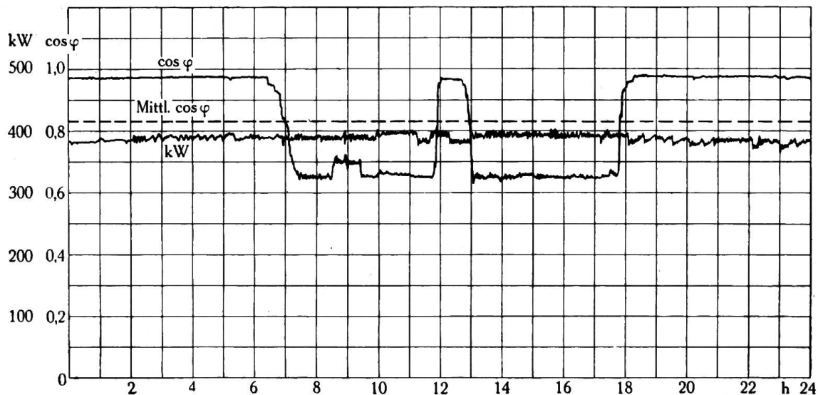
Fig. 12. Werktagsdiagramm eines grösseren Fabrikunternehmens. Wegen der Heizkörper und Boiler ist der Leistungsfaktor nachtsüber und über die Mittagspause = 0,98. Mittlerer Leistungsfaktor 0,827.
