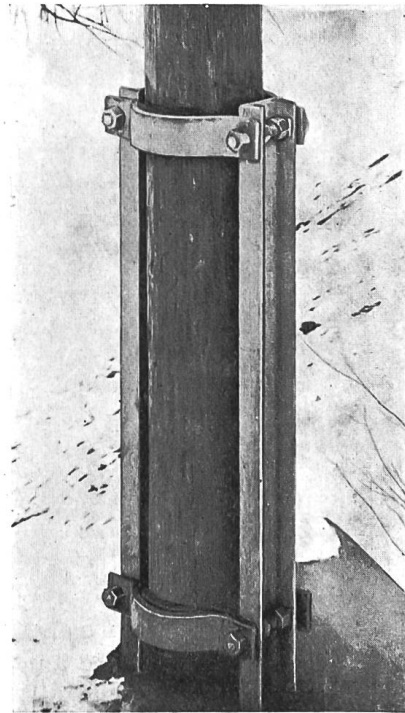
Fig. 3. Gubler -Sockel
