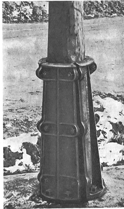
Fig. 2. Bülsterli-Sockel
