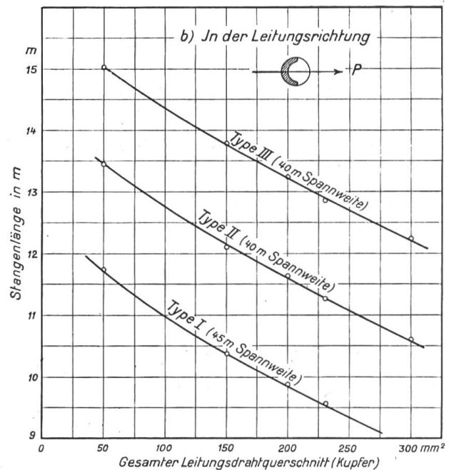
Fig. 13b. Grenzweite der Verwendbarkeit der Stangensockel „Universal“.
