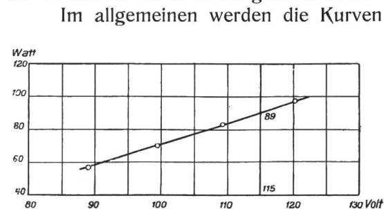
Abbildung 14. Ankerverlust bei Leerlauf in Abhängigkeit von der elektromotorischen Kraft für normale Bürsten in der Mitte der neutralen Zone.
