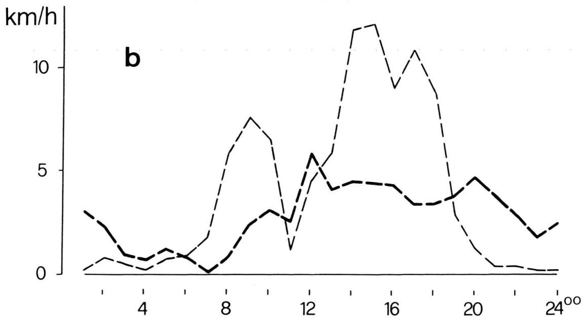
Abb. 2: Tagesgang von Lufttemperatur (a) und Windgeschwindigkeit (b) (Windschreiber nach Woelfle, Firma Lambrecht, Göttingen) in Lärchenkronen am 9. April 1969:
