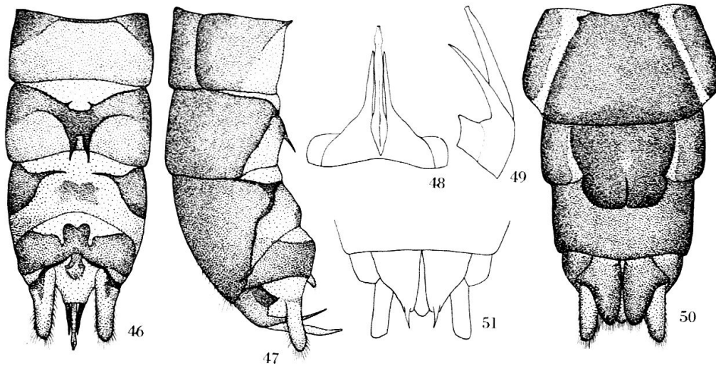
Fig. 46 à 51. Leuctra ligurica n. sp. — 46. Abdomen du ♂, face dorsale. — 47. Id. de profil. — 48. Specillum et paraproctes du ♂, face ventrale. — 49. Id., de profil. — 50. Abdomen de la ♀, face ventrale. — 51. ♀ à paraproctes anormaux.
