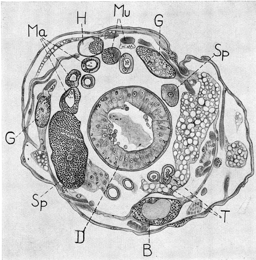
Abb. 12. Querschnitt durch eine Tineola -Raupe (B: Bauchganglion, D: Darm, G: Gonaden, H: Herzschauch, Ma: Malpighische Gefäße, Mu: Muskulatur, Sp: Spinnndrüsen, T: Tracheen; alle diese Organe sind mit Sporen verseucht).
