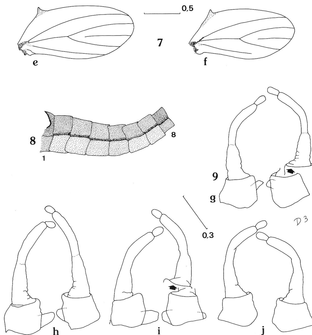
Figs 7 - 9. Imagos mâles de Baetis oukaimeden THOMAS & SARTORI n. sp. Echelle en mm. 7: aile postérieure chez deux individus (e et f). 8: abdomen en vue latérale. 9: genitalia ♂ en vue ventrale, chez quatre individus (g, h, i, j).
