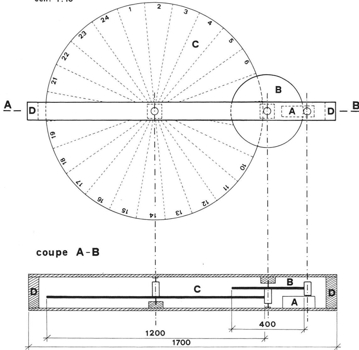
Fig. 1: Plan de l'appareil construit pour enregistrer les sorties de larves: l'axe d'un petit moteur électrique (A) à courant continu, actionne par friction un disque de démultiplication (B) fixé dans la charpente de l'appareil (D). Le disque englué (C) de 120 cm de diamètre divisé en 24 portions, appuie sur l'axe du disque de démultiplication. Un redresseur de courant et un transformateur à voltage réglable permettent de régler sa vitesse de rotation.
