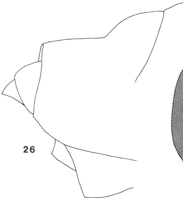
Fig. 24-26. Extrémité de l'abdomen de ♀♀ Paragus , de profil. - 24. quadrfasciatus . - 25. bicolor . - 26. cinctus .
