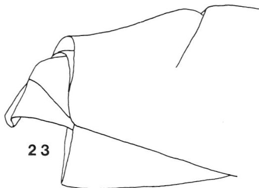
Fig. 16-23. Extrémité de l'abdomen de ♀♀ Paragus , de profil. - 16. strigatus . - 17. albifrons . - 18. flammeus . - 19. absidatus . - 20. compeditus . - 21. finitimus . - 22. majoranae . - 23. punctulatus .
