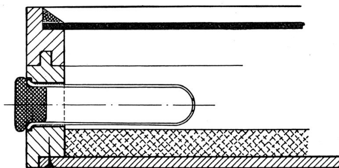
Fig. 1. — Schnitt durch die Vorderwand eines hölzernen Insektenkastens mit eingebauter Giftschleuse.
