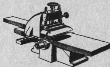
Abrihtmaschine mit Dickehobelapparat
