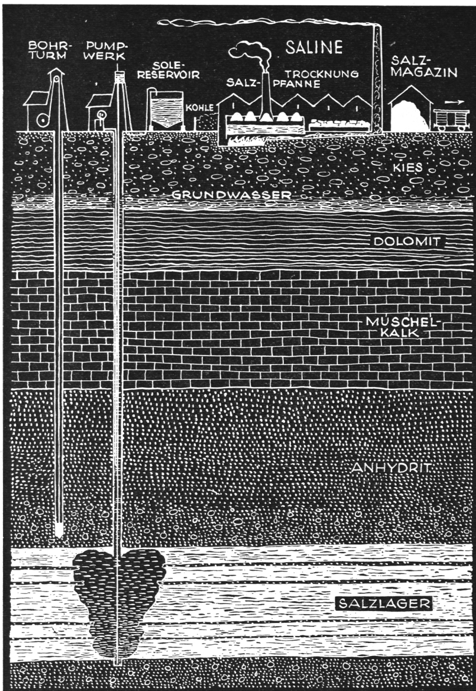
Querschnitt durch das Salzager von Schweizerhalle mit Saline um 1940.
