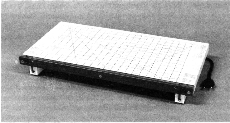
Kunststoff-Biegeapparat PA 3750 mit integriertem Netzgerät, Biegelänge 400 mm
